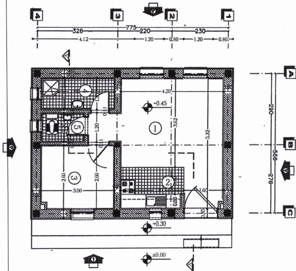
احداث ساختمان سرایداری ۵۴/۵ مترمربع
