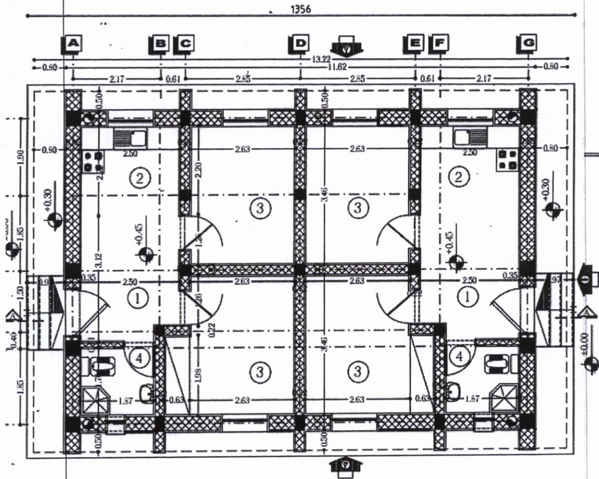
احداث ساختمان منزل پزشک ۱۱۷ مترمربع
