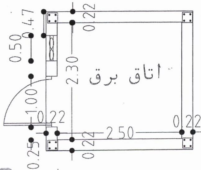
احداث ساختمان اتاق برق ۸ مترمربع
